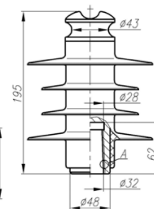
ШСК 12,5-10-4 УХЛ1 исполнение 1
