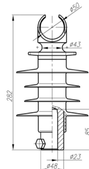
ШСК 12,5-10-4 УХЛ1 исполнение 3
