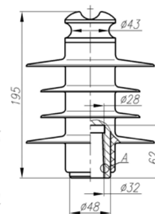
ШСК 12,5-20-4 УХЛ1 исполнение 1
