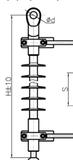
Исполнение СП (Серьга/Пестик)
