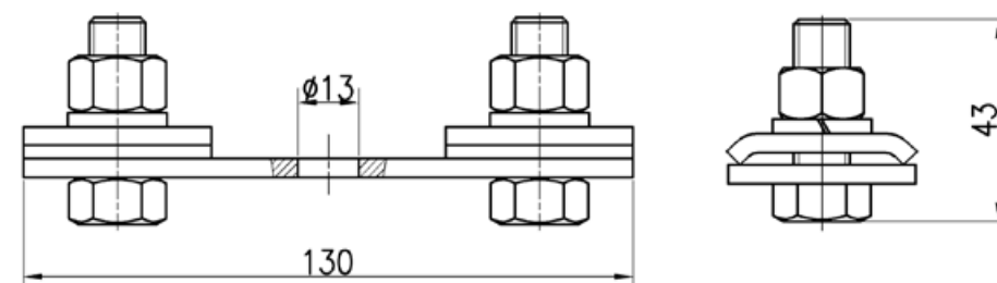
Планка для изоляторов ПСКр 9/800-60
