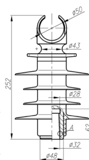
ШСК 12,5-20-4 УХЛ1 исполнение 3
