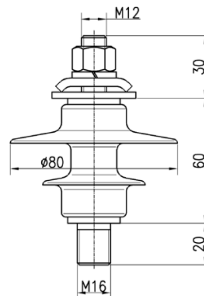
ПСКр 9/800-60-А-VII
