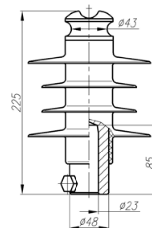
ШСК 12,5-10-4 УХЛ1 исполнение 3
