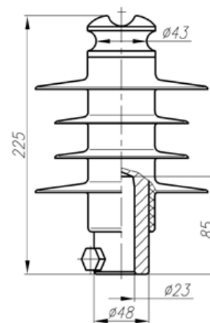
ШСК 12,5-20-4 УХЛ1 исполнение 2
