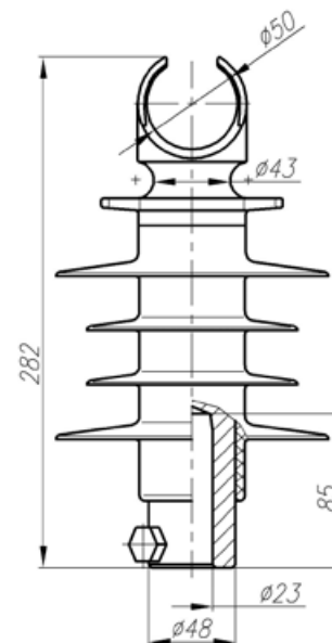
ШСК 12,5-20-4 УХЛ1 исполнение 2
